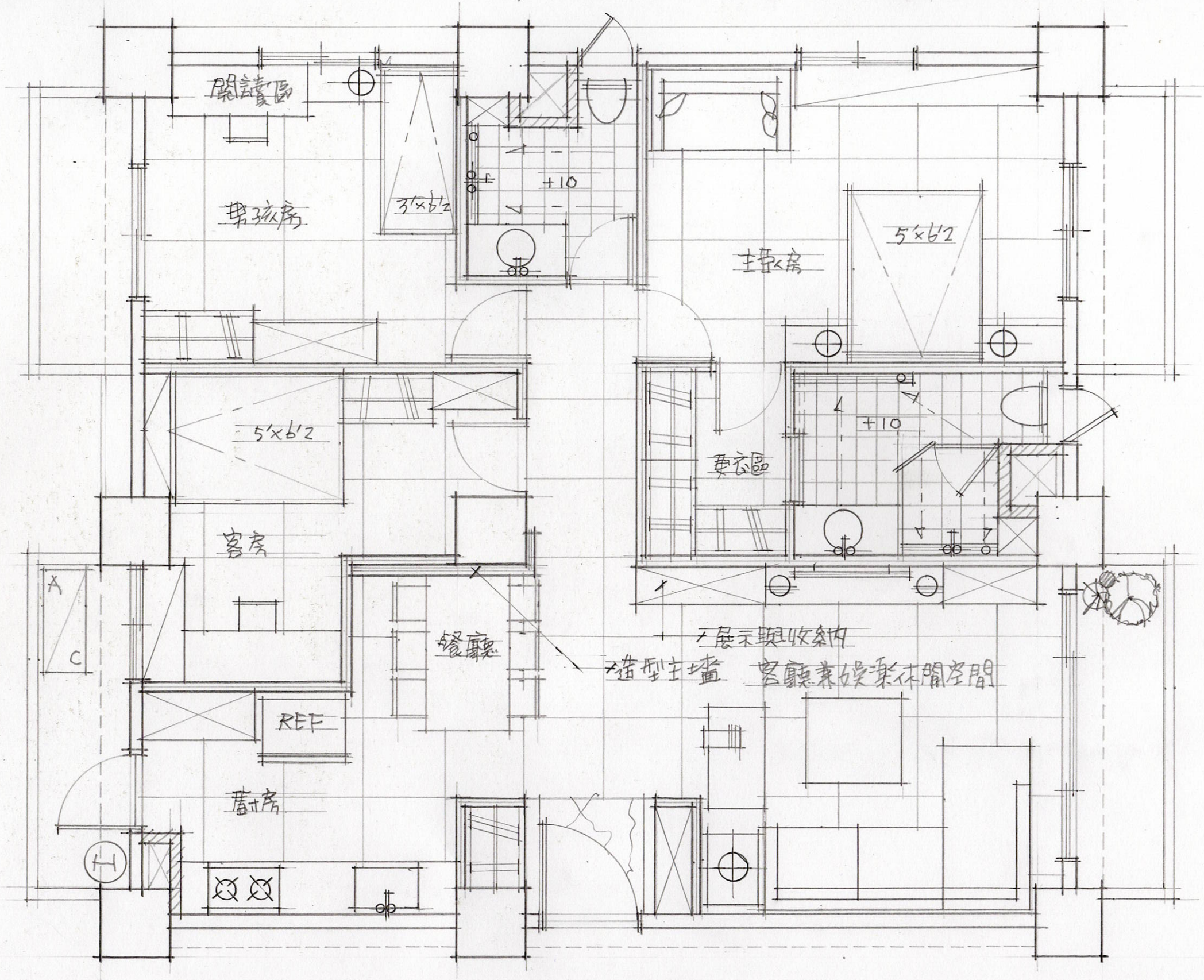
201 D 平面配置圖 比例 1/50
