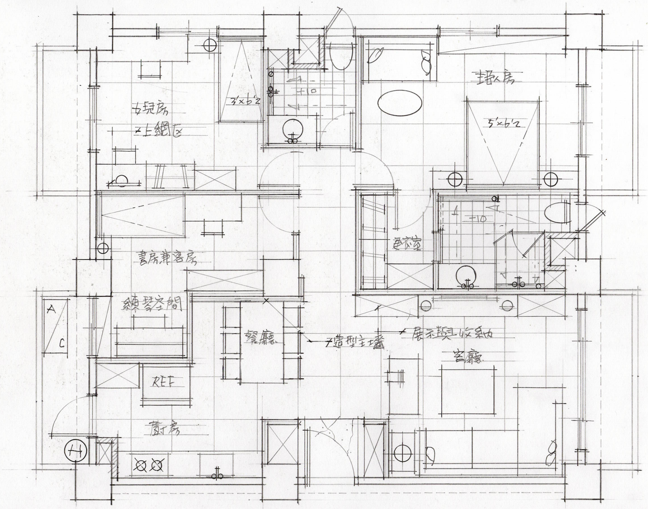
201C 平面配置圖 比例: 1/50
